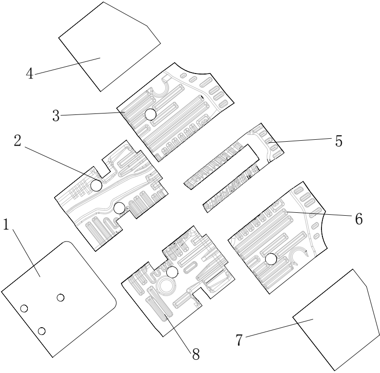
图一 地板隔热垫分解图
